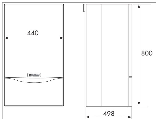
Obr. 3.6: Rozměry kotle
